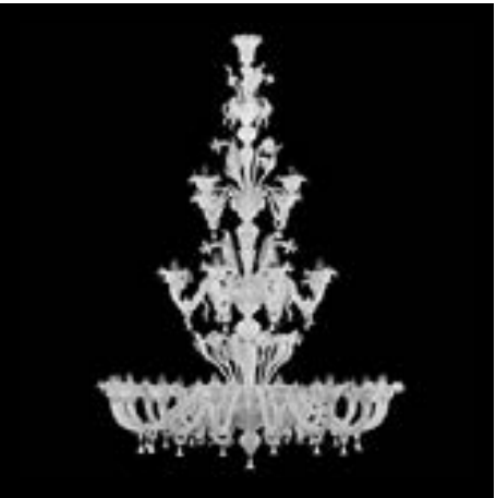
S0811-16+8+4-W Ø 160 cm - H 220 cm - C 55 cm - R 14 cm E14 28 x MAX 40W 60 KG
